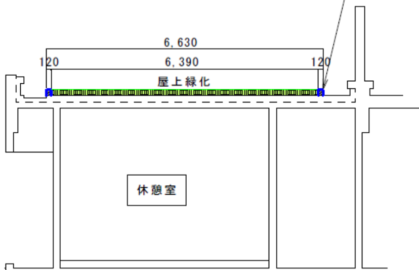
①-①断面図 S=1/100
